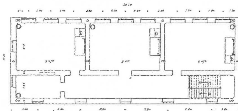
75 'Υπόδειγμα εξατάξιου διδακτηρίου, 1911, (σειρά Α) α' κάτωψη ισόγειου β' κάτωψη όρόφου γ' κάτωψη θεμελίων
