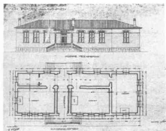
90. Μονότοξο τριτάξινο διδακτήριον, τύπος 33. 'Αρχ. Π.
