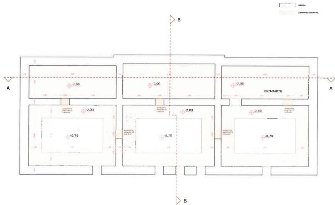
ΕΙΚΟΝΑ Γ.1.1., Σχέδιο Καθαιρέσεων, Κάτοψη Υπογείου, εκτός κλίμακας.
