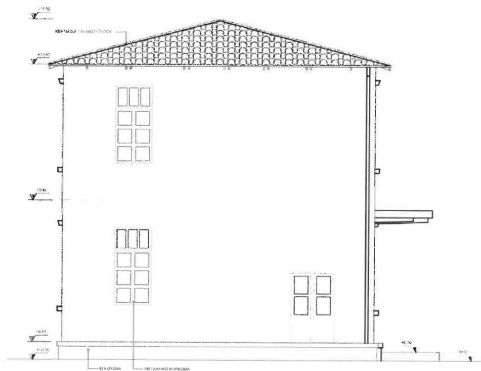
ΕΙΚΟΝΑ Β.6. Αποτύπωση υφιστάμενης κατάστασης, Όψη Β (Πλάγια) εκτός κλίμακας.
