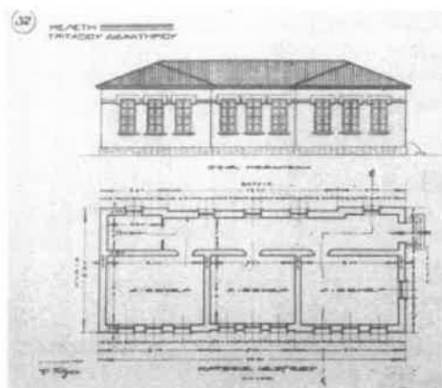
89. Μονότοξο τριτάξινο διδακτήριον, τύπος 32. 'Αρχ. Π. Σωφράν. (Πολύτρος) 1926.
