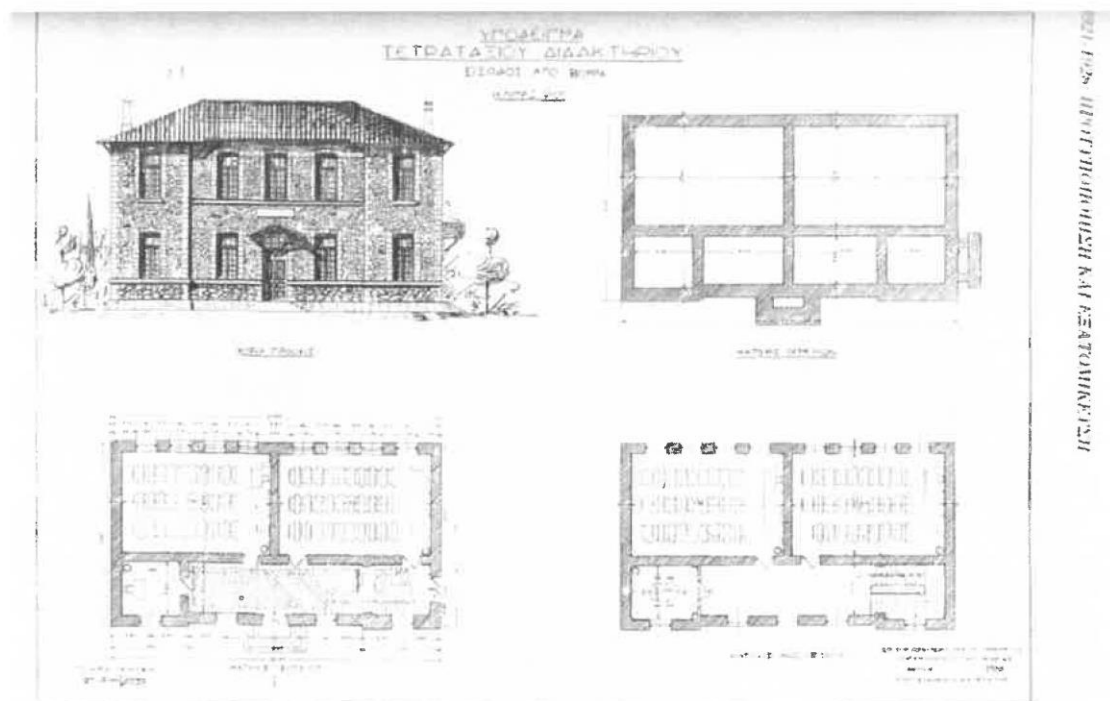
91. Υπόδειγμα τετρατάξιου διδακτηρίου, 1926.
