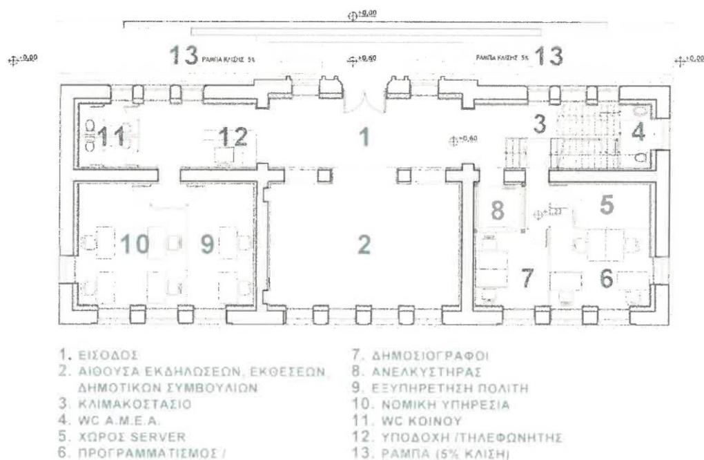
ΕΙΚΟΝΑ Γ.2.1. Πρόταση Διαρρύθμισης, Κάτοψη Ισογείου, εκτός κλίμακας.
