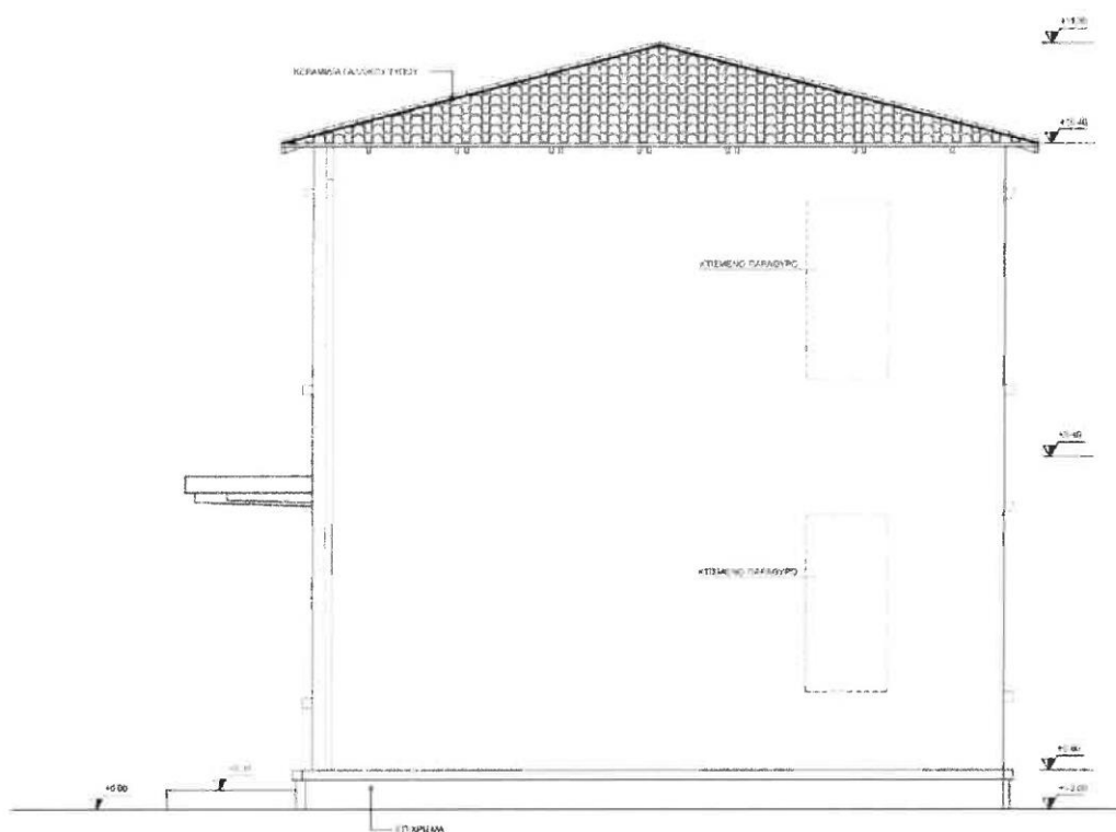
ΕΙΚΟΝΑ Β.8. Αποτύπωση υφιστάμενης κατάστασης, Όψη Δ (Πλάγια), εκτός κλίμακας.
