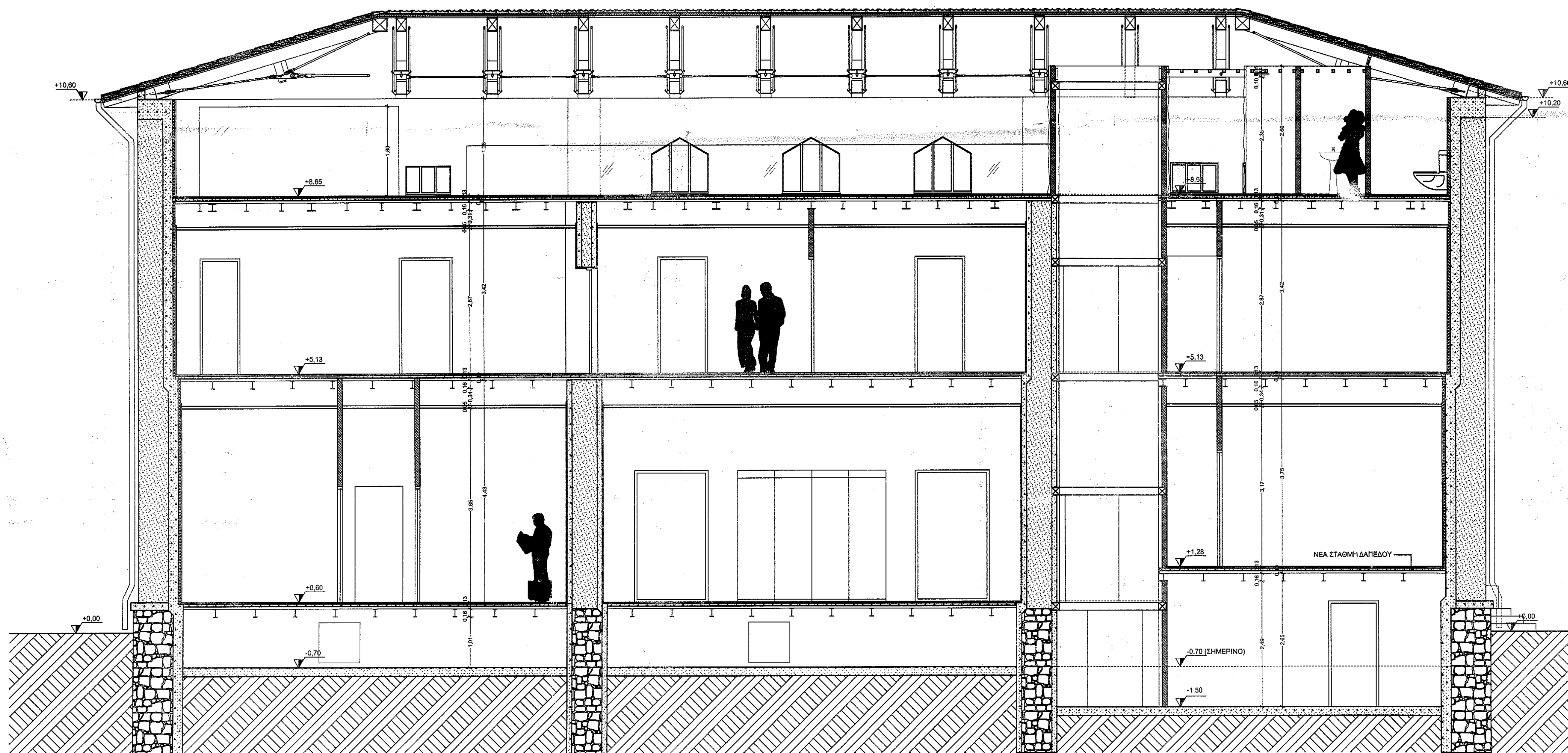
TOMH A-A
