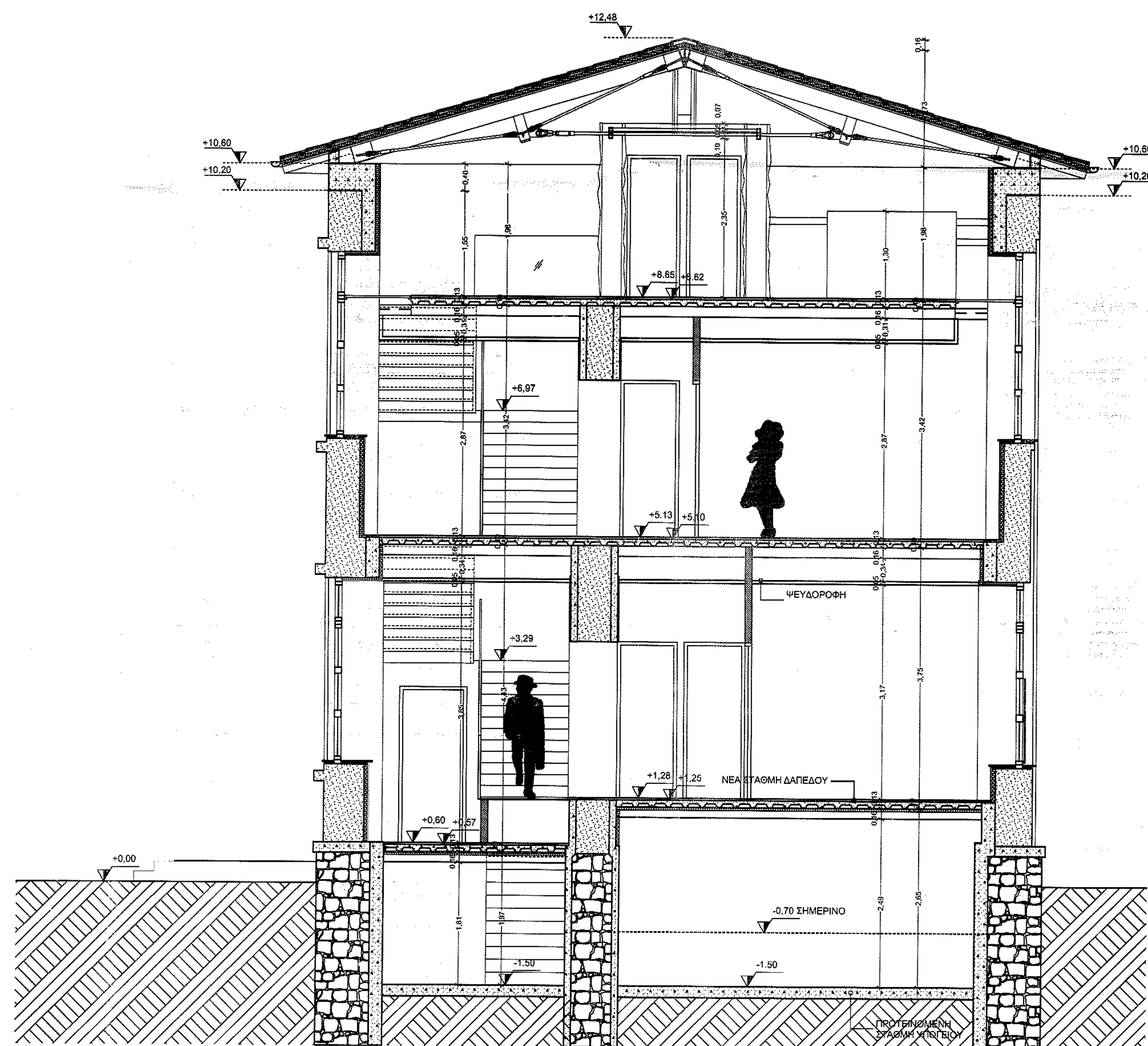
ΤΟΜΗ Β-Β
